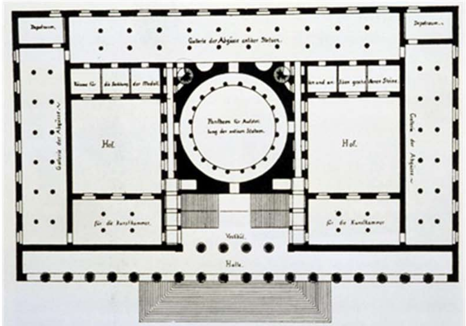
40_K_F_Schinkel_GR_1._OG_Altes_Museum_Berlin.jpg
