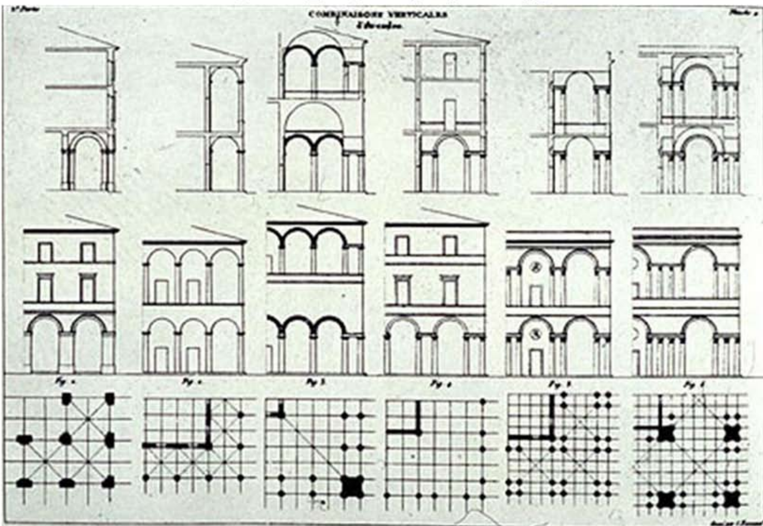
Abb. 114 Jean-Nicolas Louis Durand, Die 'Bautypen' (1823)
