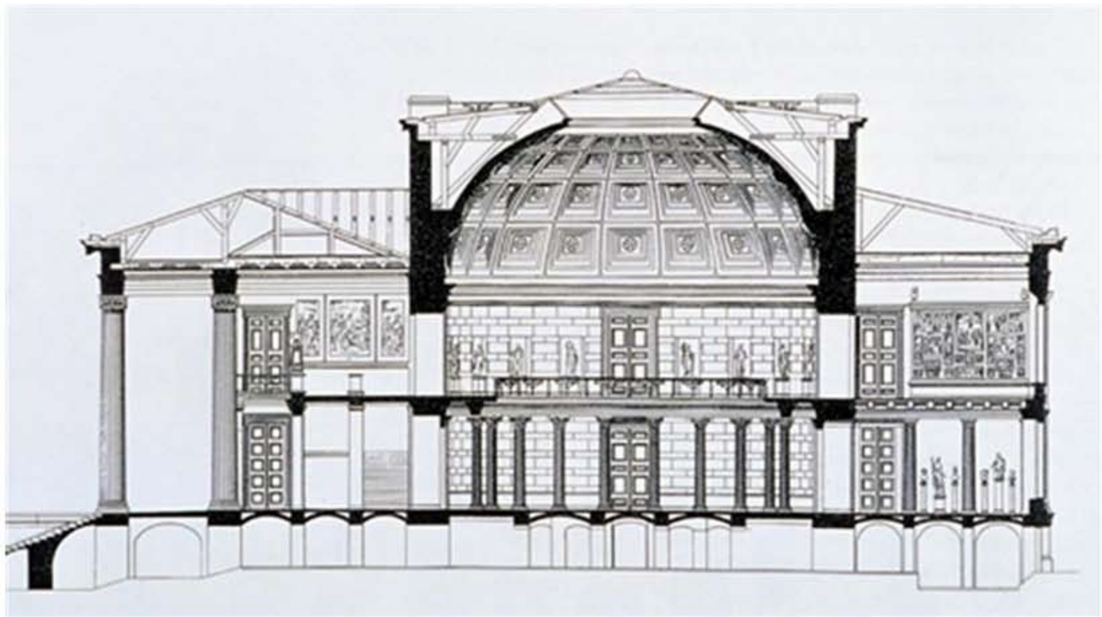
43_K_F_Schinkel_Laengsschnitt_Altes_Museum_Berlin.jpg
