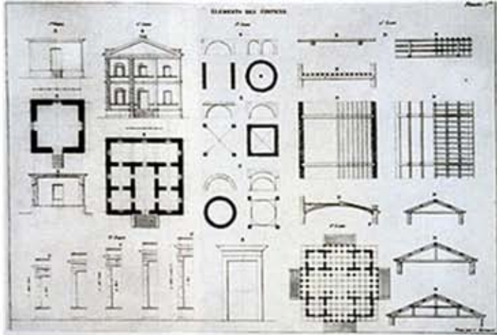
Abb. 113 Jean-Nicolas Louis Durand (1760-1834), die 'Baulemente' (1823)
