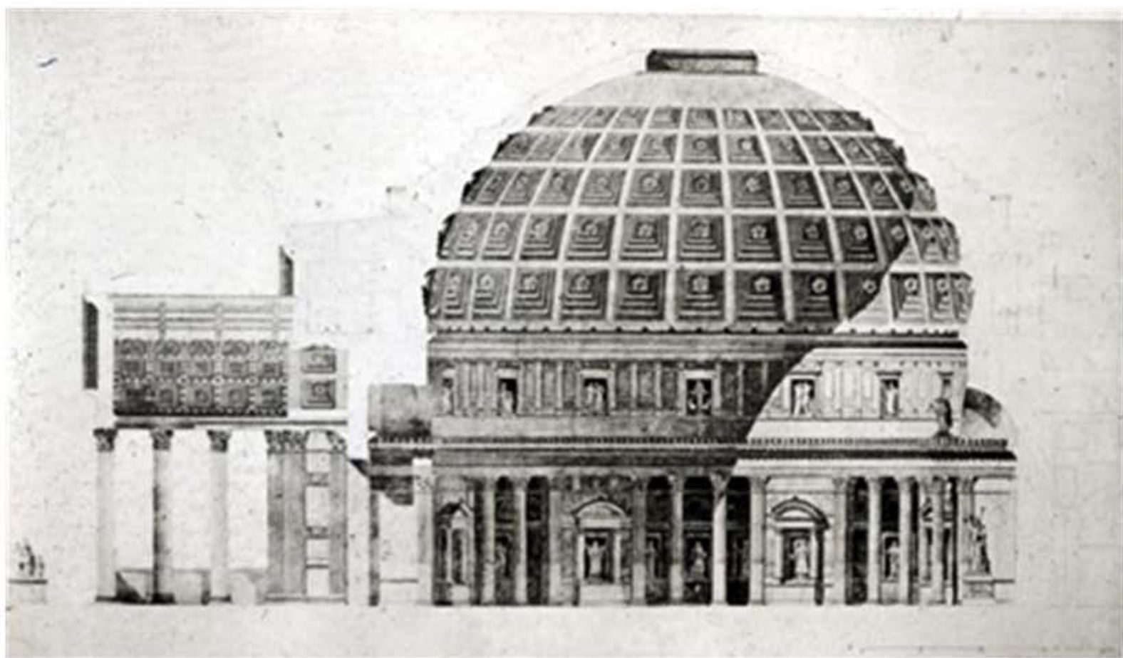
44_Schnitt_durch_das_Pantheon_Rom.jpg
