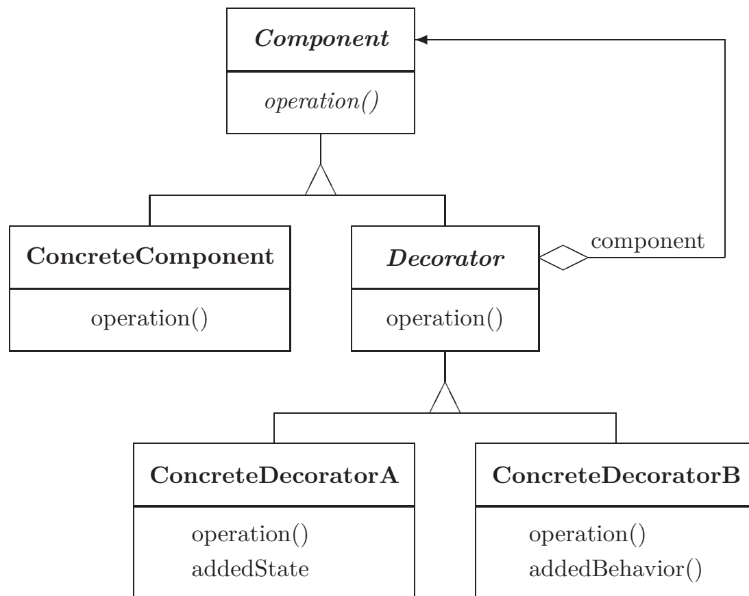
Abbildung 5.2.: Struktur von Decorator
