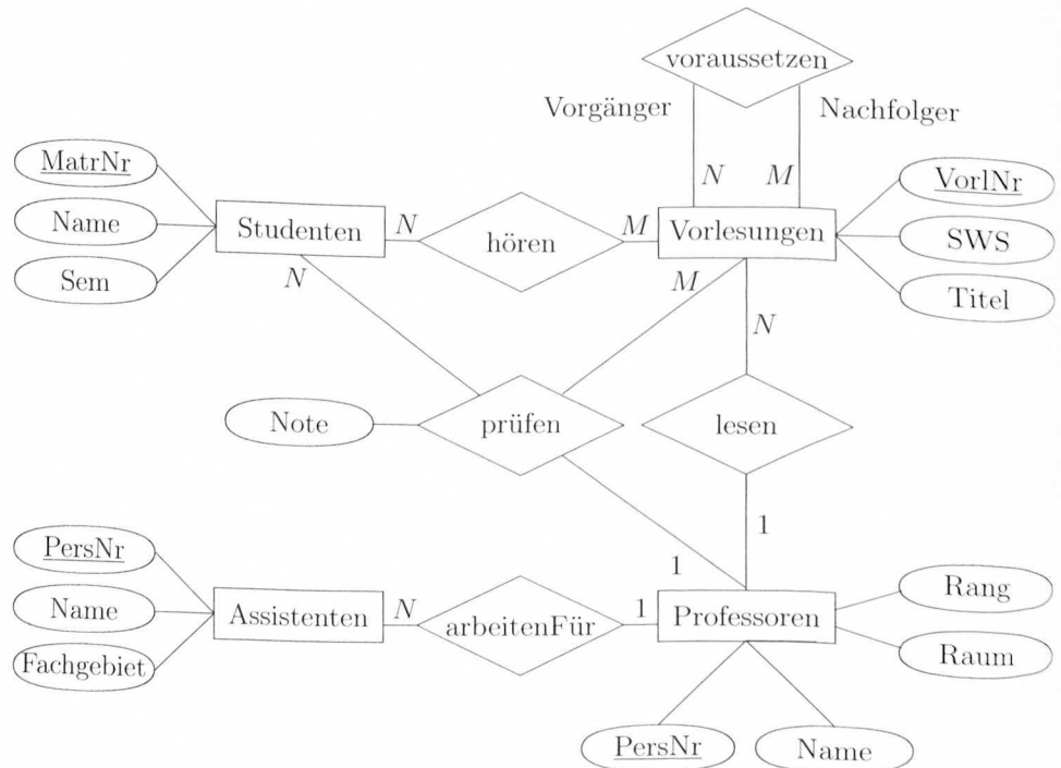
Abbildung 2.7: Markierung der Funktionalitäten im Universitätsschema
