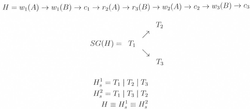
Abbildung 11.10: Serialisierbare Historie H mit zugehörigem Serialisierbarkeitsgraphen SG(H) und den zwei äquivalenten seriellen Historien H_s^1 und H_s^2 .
