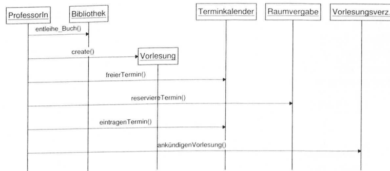
Abbildung 2.29: Das UML-Interaktionsdiagramm zur Planung einer neuen Vorlesung
