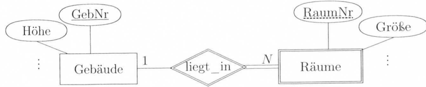
Abbildung 2.11: Ein existenzabhängiger (schwacher) Entitytyp
