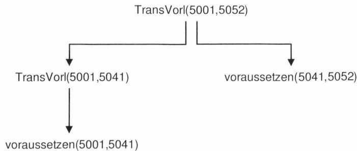
Abbildung 4.6: Herleitung eines Tupels der Sicht TransVorl
