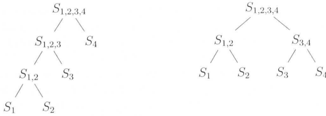
Abbildung 2.18: Mögliche Konsolidierungsbäume zur Herleitung des globalen Schemas S_{1,2,3,4} aus 4 Teilschemata S_1, S_2, S_3 und S_4 : links ein maximal hoher und rechts ein minimal hoher Konsolidierungsbaum
