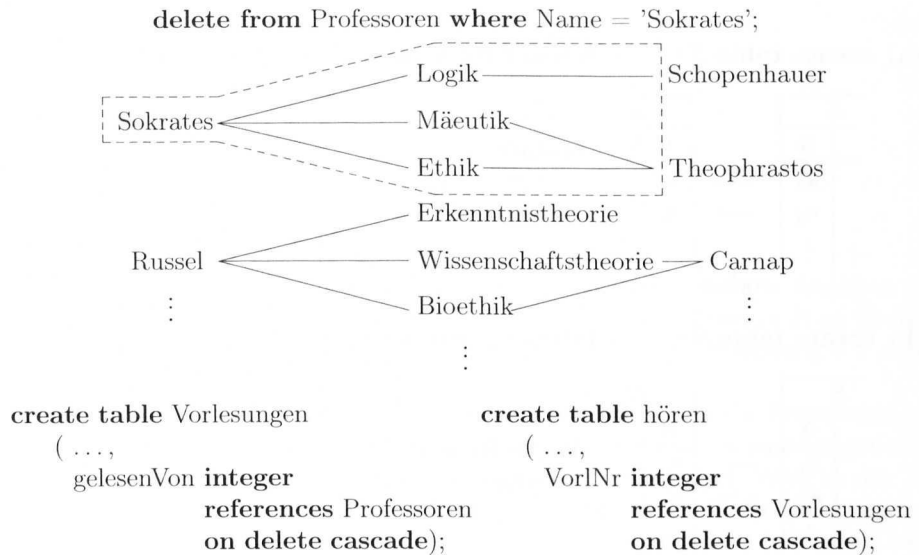
Abbildung 5.3: Kaskadierende Löschoperationen
