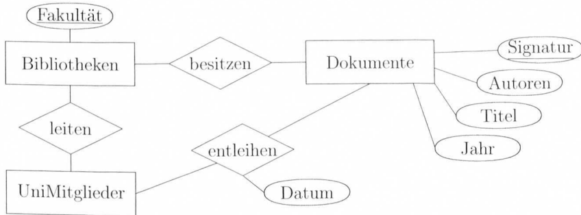
Sicht 2: Bibliotheksverwaltung
