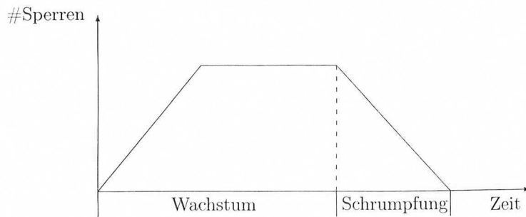
Abbildung 11.14: Zwei-Phasen Sperrprotokoll
