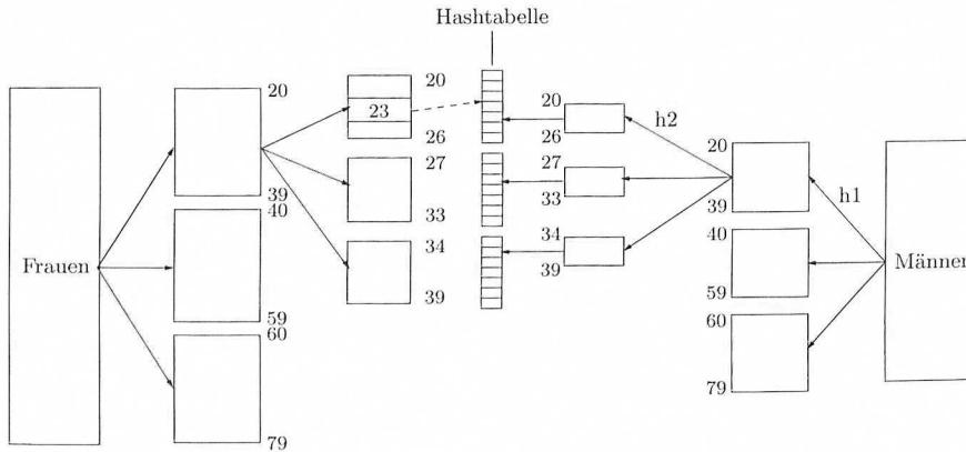
Abbildung 8.24: Berechnung von Frauen \bowtie_{Frauen.Alter=Männer.Alter} Männer
