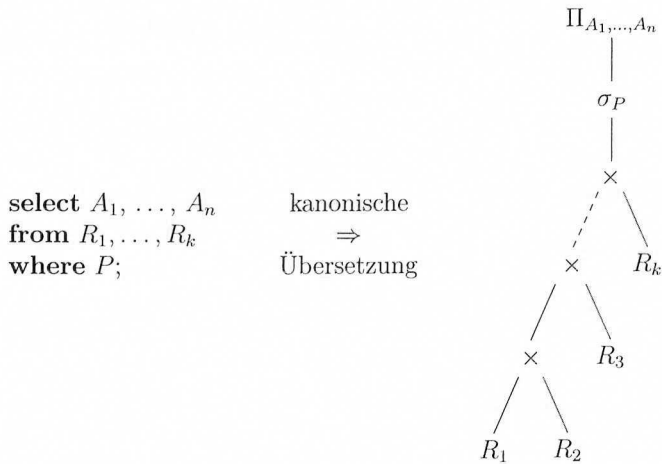
Abbildung 8.2: Kanonische Übersetzung einer SQL-Anfrage
