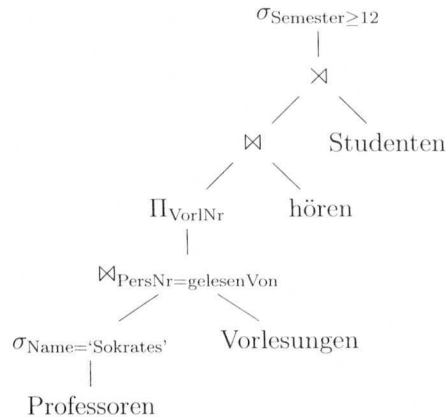
Abbildung 3.10: Baumdarstellung des Algebra-Ausdrucks
