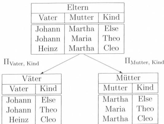
Abbildung 6.2: Verlustlose Zerlegung der Relation Eltern
