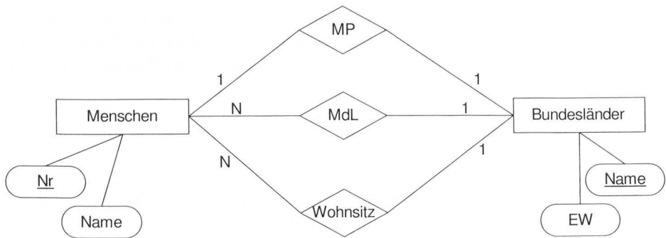
Abbildung 3.6: Beziehungen zwischen Menschen und Bundesländern
