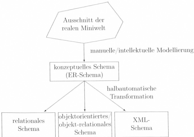
Abbildung 1.2: Übersicht der Datenmodellierung
