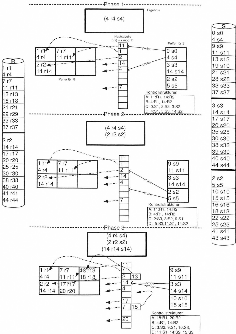
Abbildung 8.29: Die ersten drei Phasen des G-Joins
