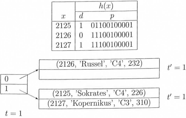
Abbildung 7.25: Ein Hash-Index
