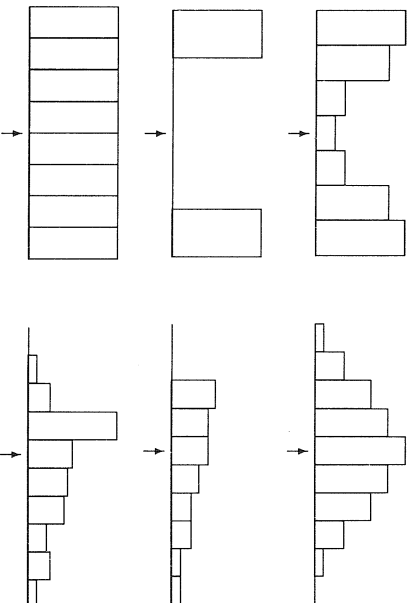
Abbildung 3.6: Verschiedene Verteilungen bei gleichem Mittel.
