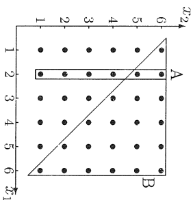
Abbildung 4.2: Bedingte Ereignisse.
