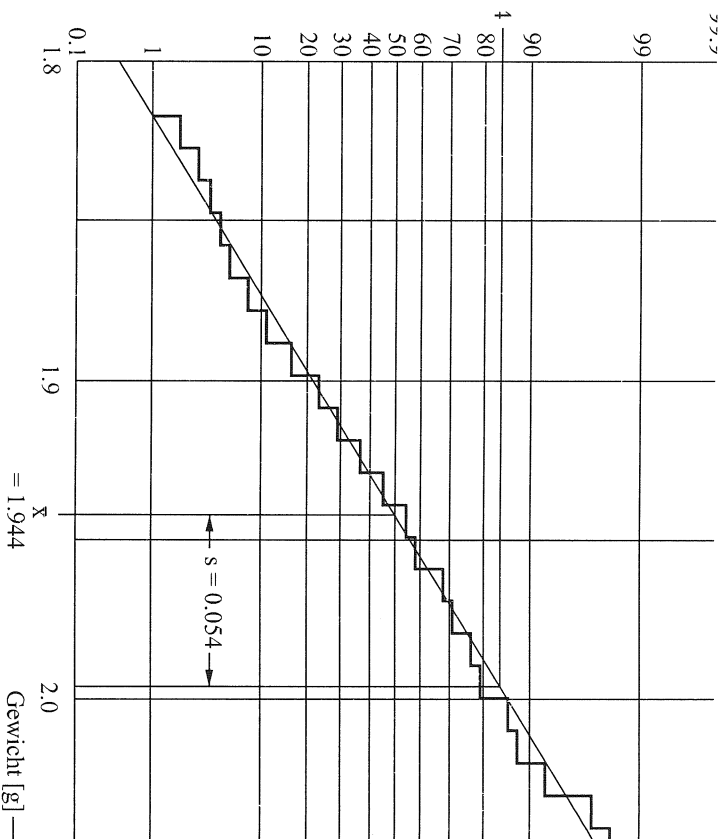
Abbildung 4.9: Wahrscheinlichkeitspapier.
